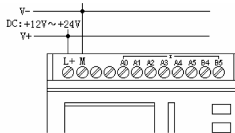
Рис.2.7 DC-тип
