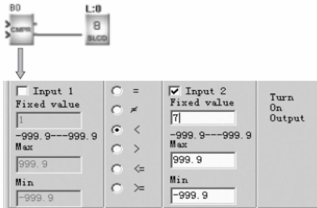
Рис.4.3 Установка свойств аналогового блока сравнения.
