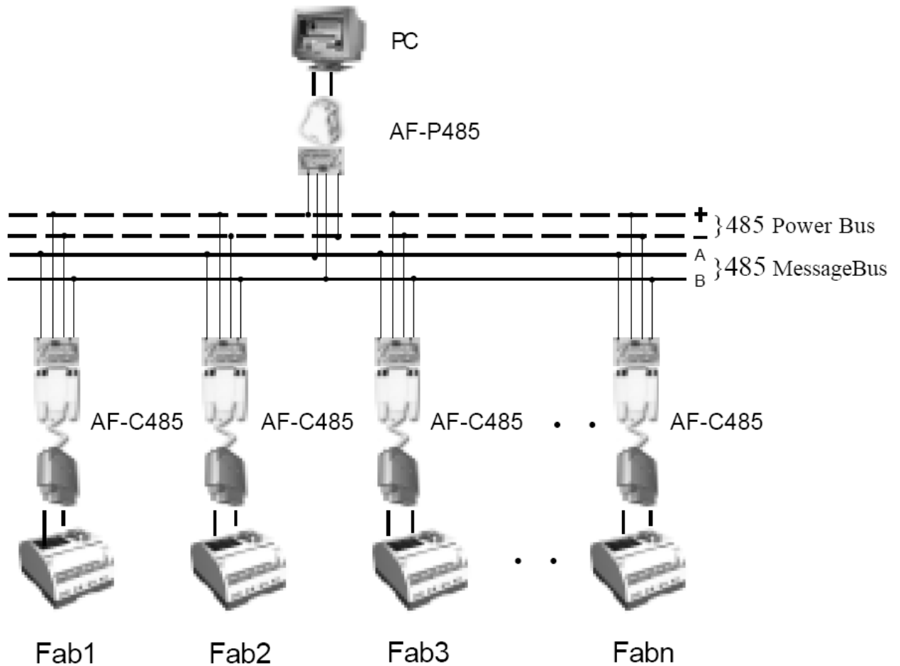
Рис. 2.12 Способ подключения
